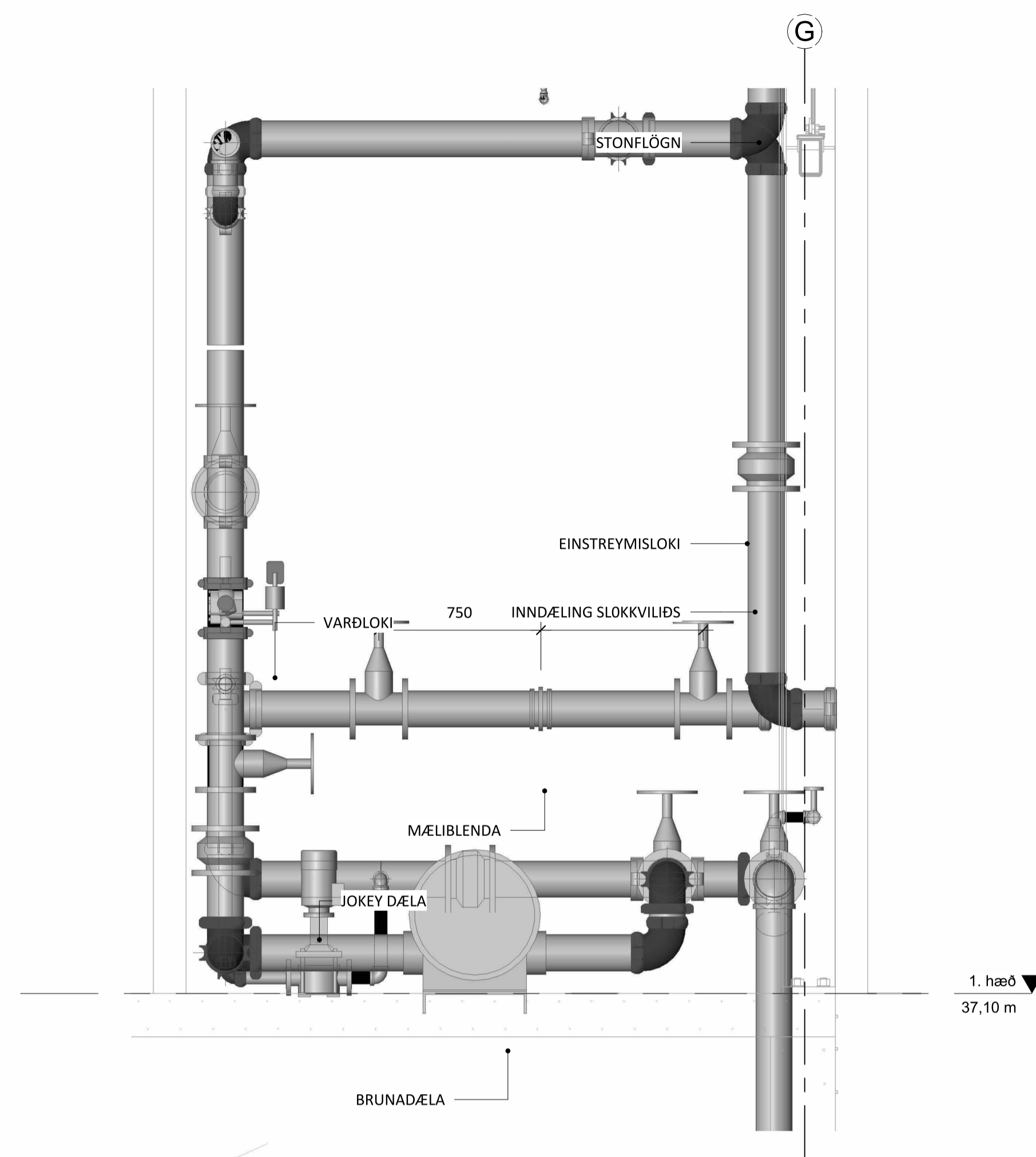
5-5 SNID Í MÆLIBLENDU 1 : 20
